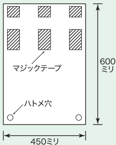
仕様図(裏面)
