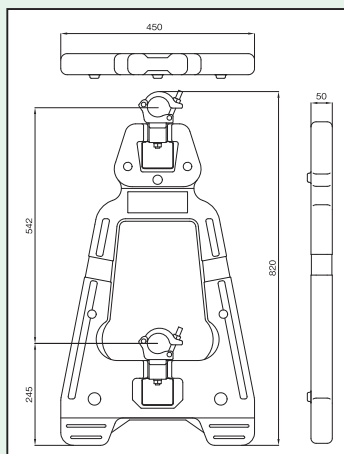
33-344 バリケード頑張郎 KYライン用(樹脂製) 33-345 バリケード頑張郎 単管パイプ兼用(金属製)
